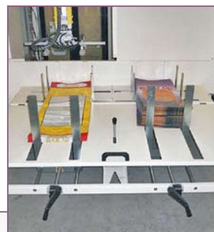
CSA 90 Almacén de sacos vacíos Standard empty sacks tray (double)
